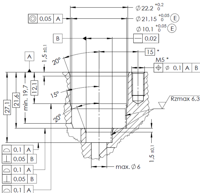
Schnittstellengeometrie P21 interface geometry P21
